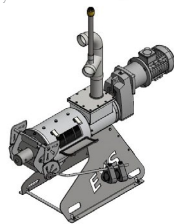
Montage mit Optionalen Zubehören Mounting with Optional Accesories
