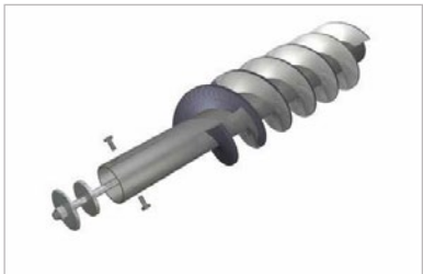
Einfache Montage der Pressschnecke und Siebe Easy montage of the Screw and screen
