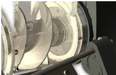
Trennung zwischen Schnecke und Getriebe Separation between body and transmission unit
