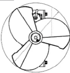
Propeller mit 3 Flügeln Propeller with 3 Blade
