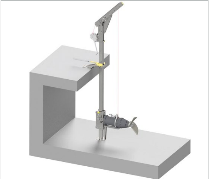
Drehbare Halterung für Vorgruben Rotatable platform positioning in biogas pits
