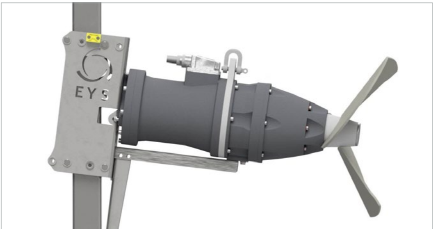
Einstellung bei stabilen Sinkschichten / -7° Bottom layer solve / -7°
